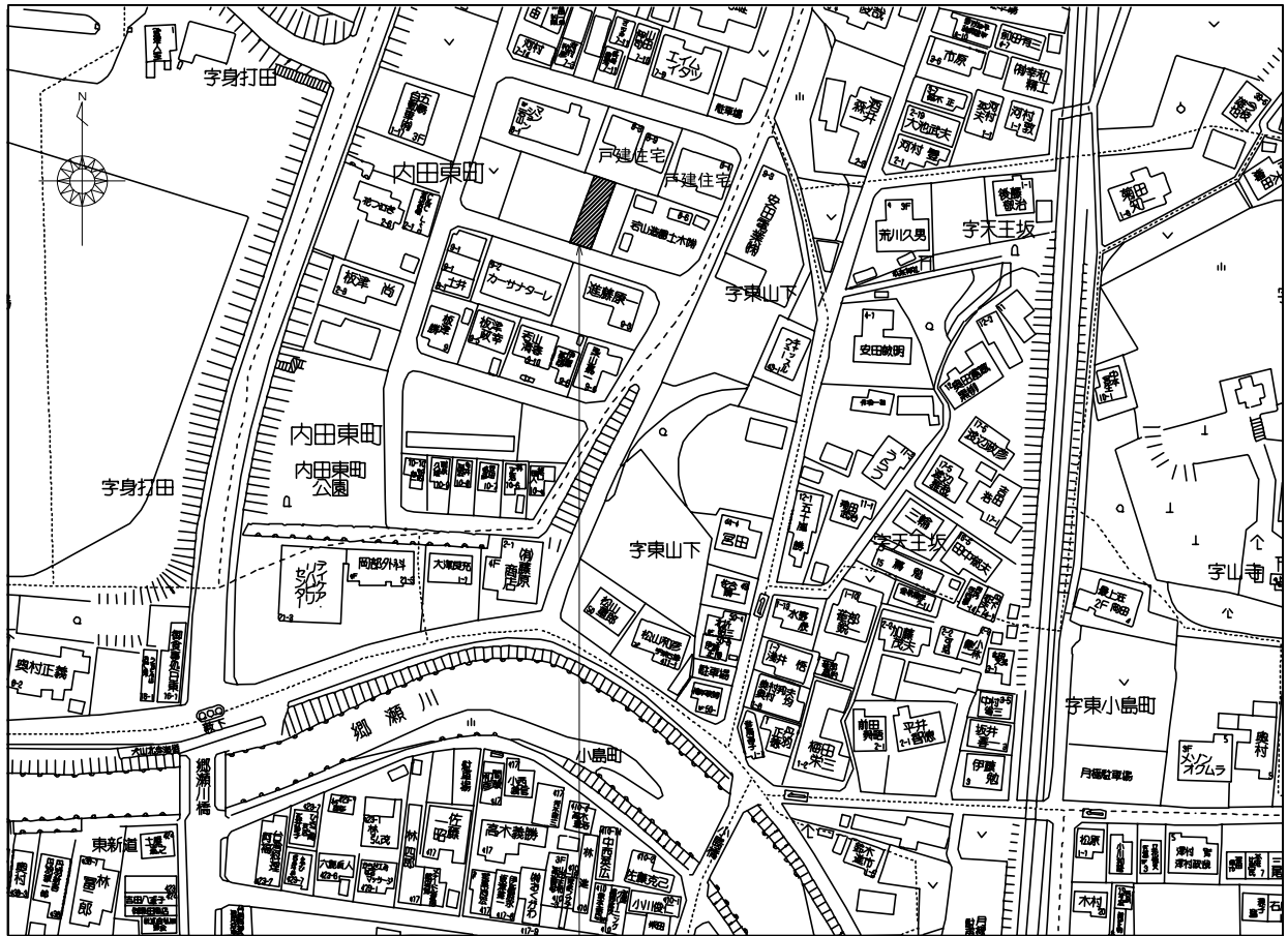
附近見取図
